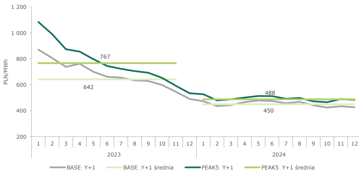
Wykres: Średnie miesięczne notowania na RTT w latach 2023–2024 (TGE). 19
