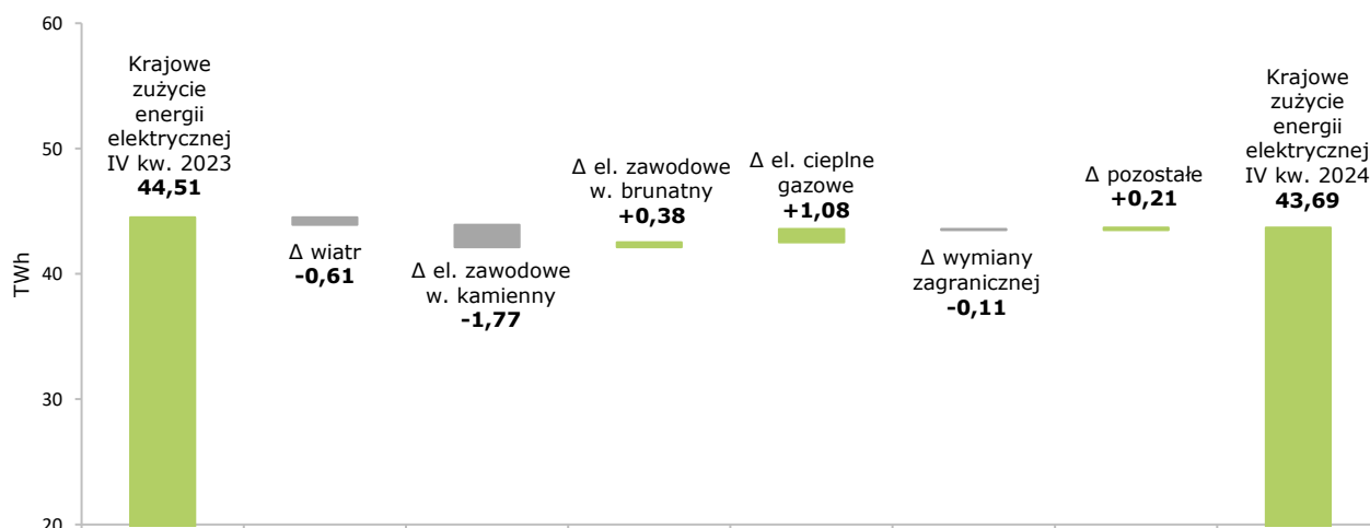
Wykres: Bilans energii w KSE w IV kwartale 2024 roku (TWh).
